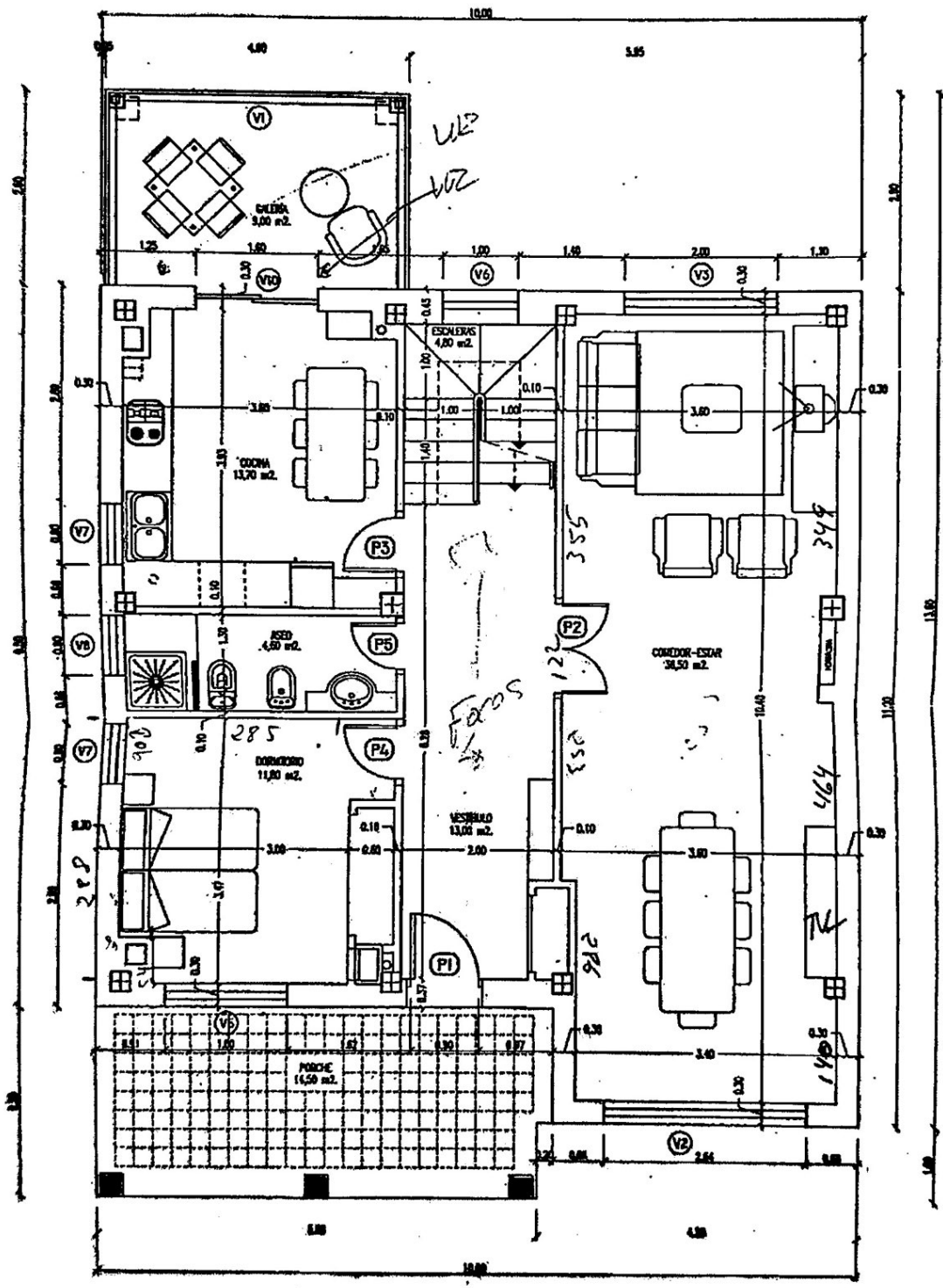
PLANTA BAJA
